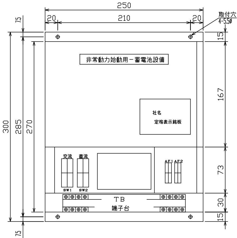
端子台配列
